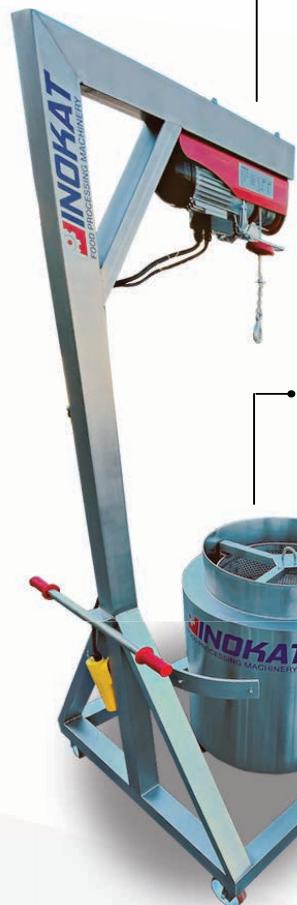
ΤΡΟΧΗΛΑΤΟ ΠΑΛΑΓΚΟ Wheeled Basket Hoist
